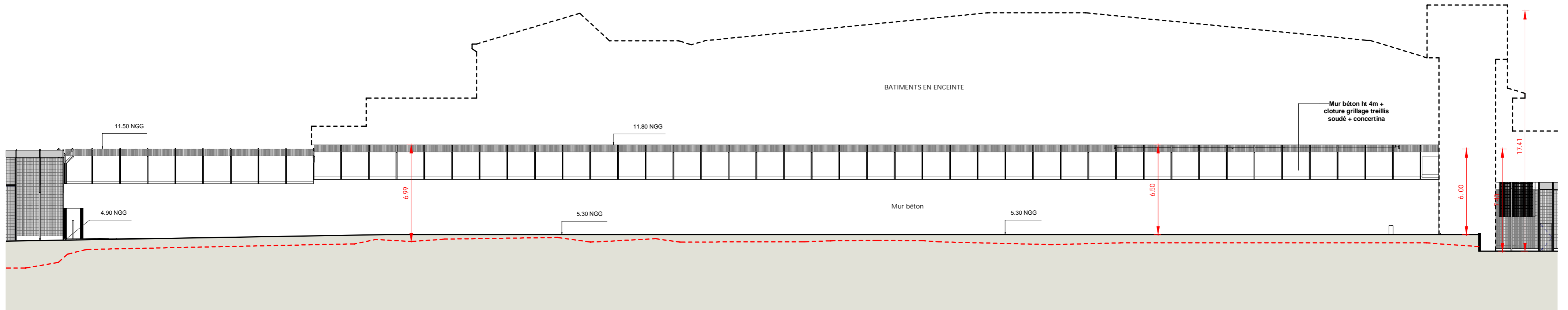
1 Elévation mur d'enceinte sud 1 : 200
